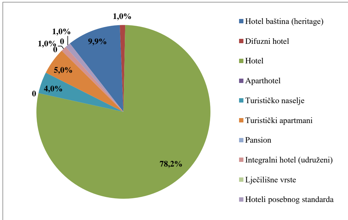
Slika 6. 1. Vrste objekta
